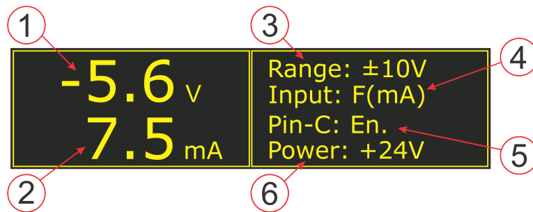
Abbildung 3: OLED Bildschirm des ValveExpert Checker 2.4 (siehe Tabelle 2 zur Erläuterung).
