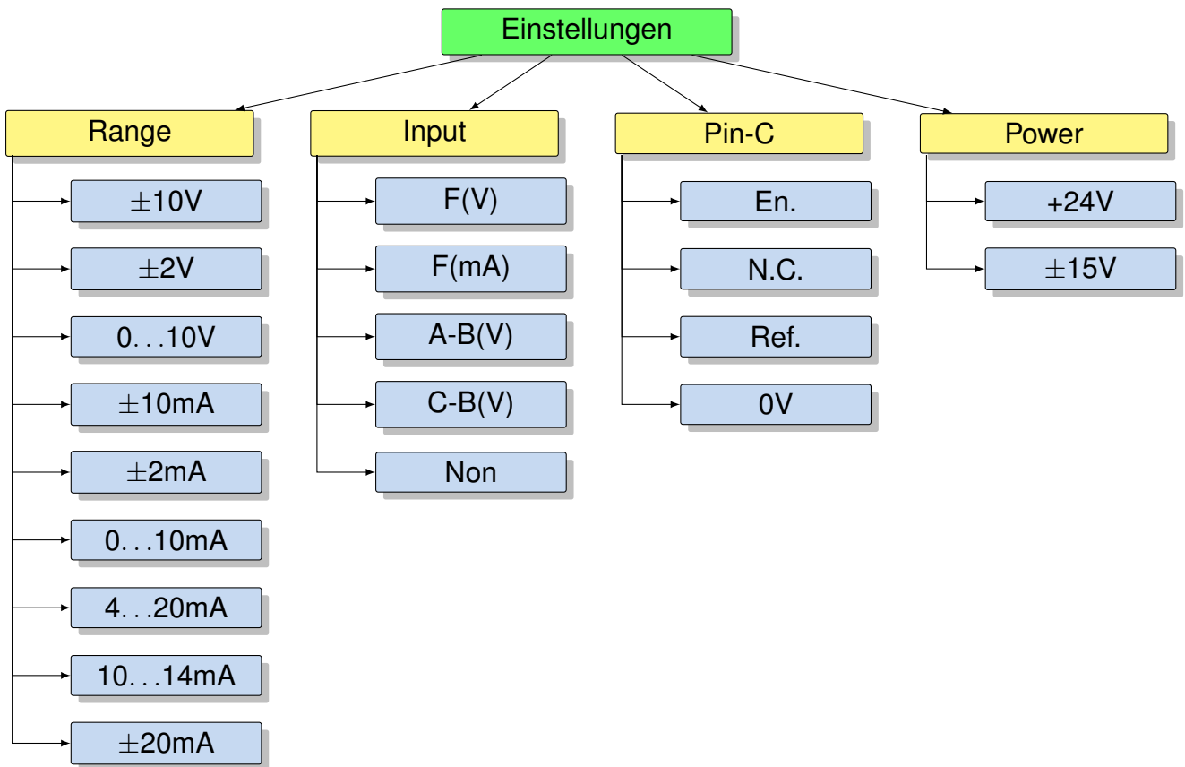
Abbildung 5: Einstellungs-Diagramm für ValveExpert Checker 2.4 (siehe Abbildung 3 und Tabelle 2).
