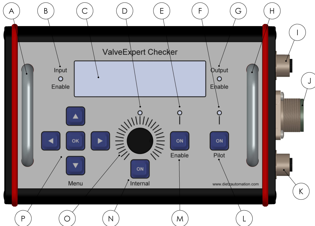
Abbildung 2: Frontplatte des Prüfgerätes ValveExpert Checker 2.4 (siehe Tabelle 1 zur Beschreibung).
